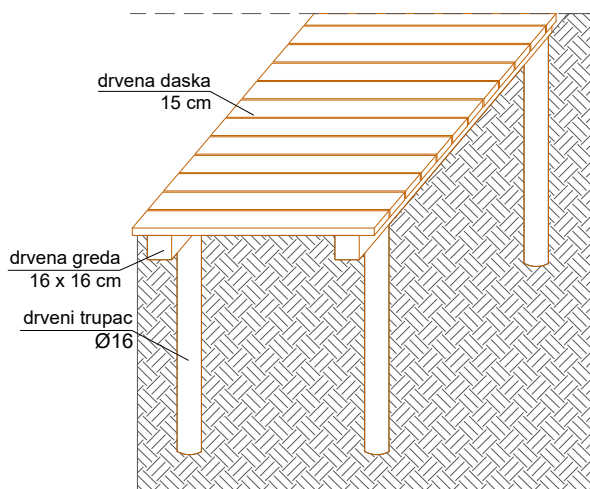
AKSONOMETRIJA STAZE
