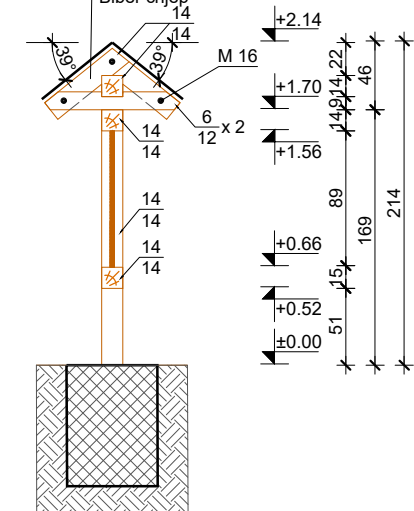
POPREČNI PRESJEK A-A
