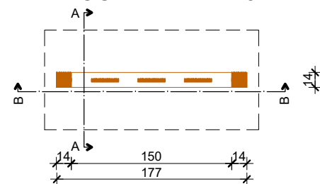
TLOCRT PRIZEMLJA
