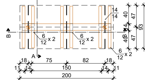
TLOCRT KROVIŠTA
