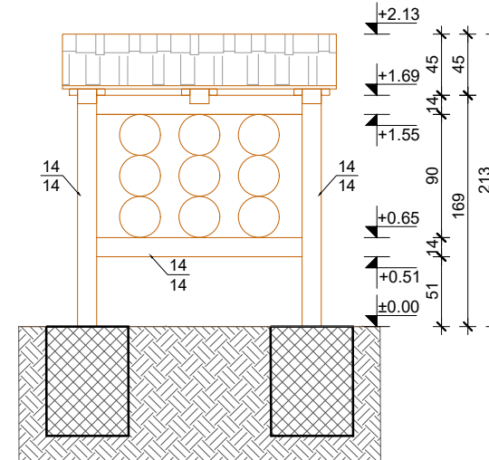
UZDUŽNI PRESJEK B-B
